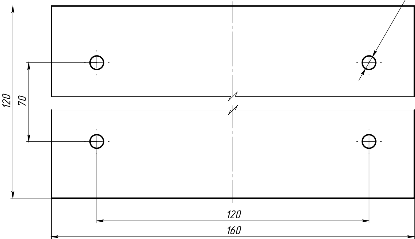
Поз.1 (Плита опорная)
